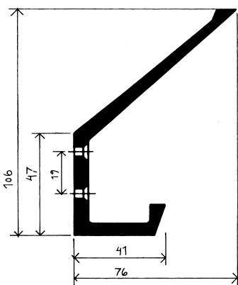
Nr 14860 dubbelkrok med synlig infästning direkt i vägg
