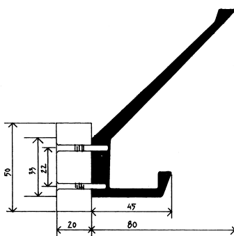
Nr 34870 dubbelkrok med dold infästning
